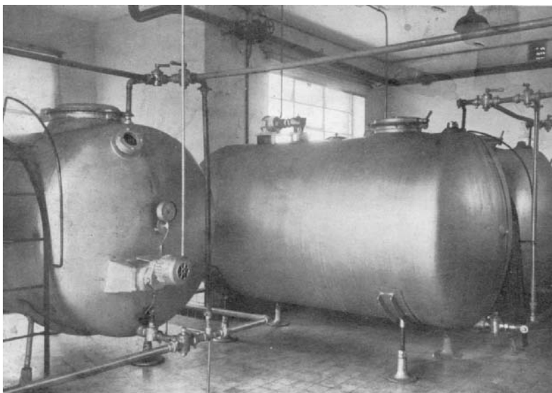
Tankenlokaal. Geïsoleerde tanks met een totale inhoud van 20.000 liter. (Fotoarchief "Het Land van Nevele")
