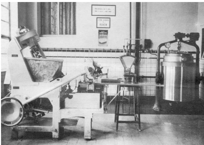
Zicht op het karnlokaal: automatische botervormmachine. Vormen, wegen en inpakken met een capaciteit van 1.200 kg per uur. (Fotoarchief "Het Land van Nevele")
