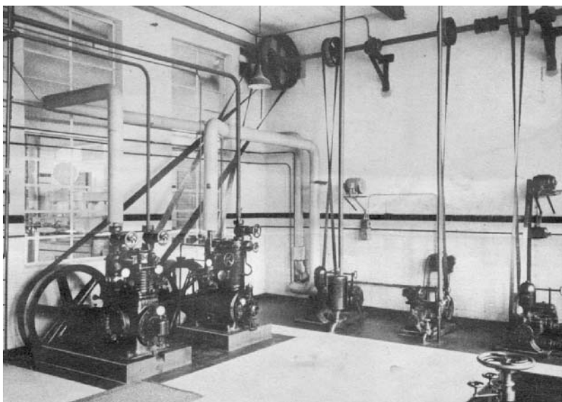
Machinekamer: ijsmachines met toebehoren voor de ijsfabricatie en diepkoeling van melk en room (Fotoarchief "Het Land van Nevele")
