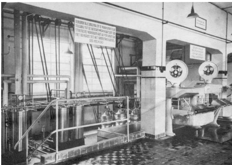
Algemeen zicht op het bewerkingslokaal van de melk. (Fotoarchief "Het Land van Nevele")
