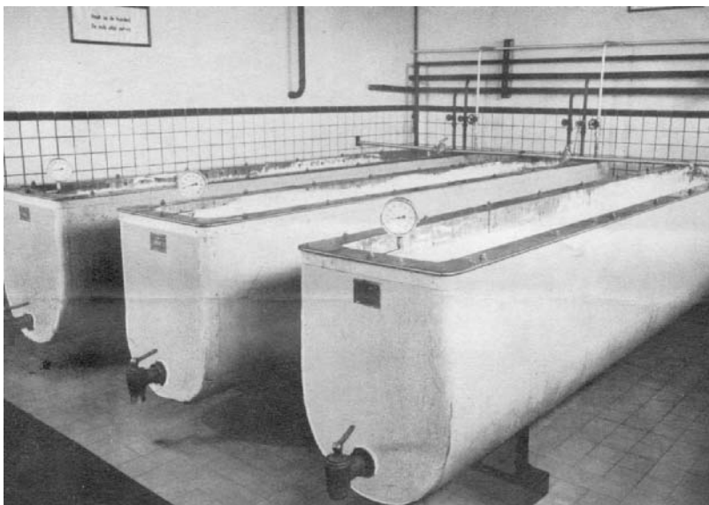
Roomrijpers met een totale inhoud van 5.000 liter. (Fotoarchief "Het Land van Nevele")
