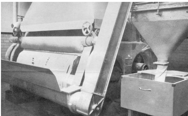
Melkpoedermachine met maalderij in volle werking, gebouw in roestvrij staal. (Fotoarchief "Het Land van Nevele")
