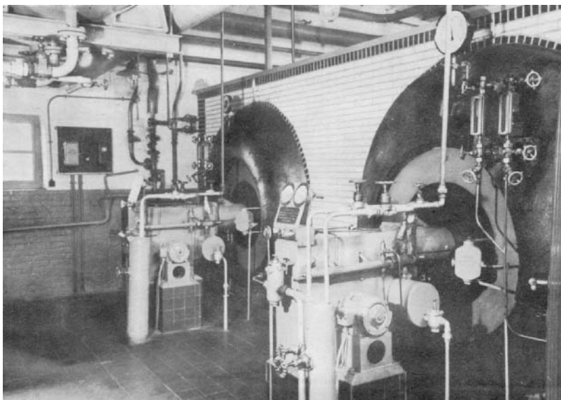
Stookinstallaties met mazoutbranders, 100 m 2 verwarmingsoppervlakte. (Fotoarchief "Het Land van Nevele")
