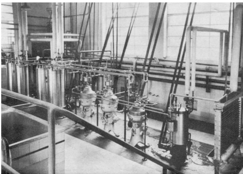
Ontromingsafdeling met pasteurisatietoestellen en koelapparaten. Verwerking: 10.000 liter melk per uur. (Fotoarchief "Het Land van Nevele")
