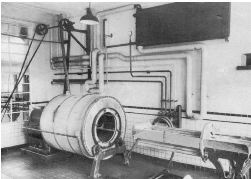
Karnkneder met een inhoud van 3.600 liter. (Fotoarchief "Het Land van Nevele")
