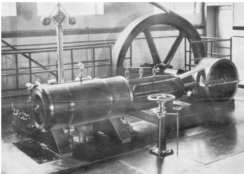
Moderne stoommachine, aandrijving 100 pk. (Fotoarchief "Het Land van Nevele")
